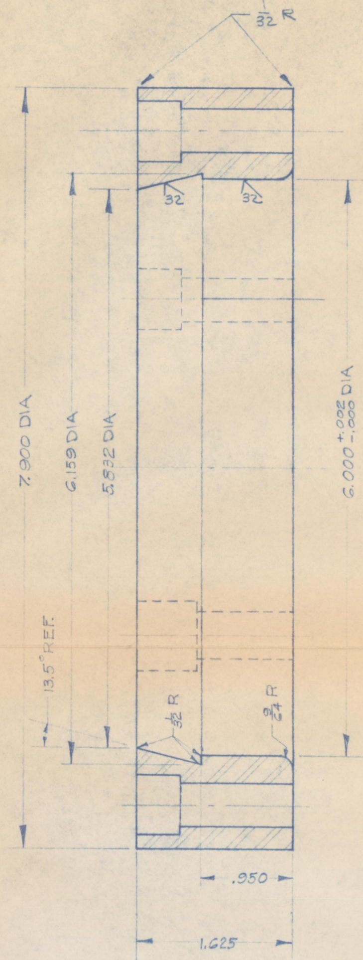
SECTION A-A
